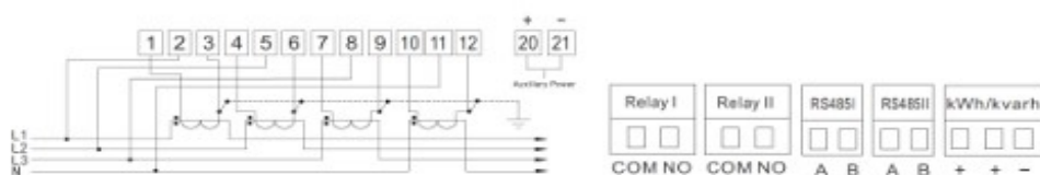
Připojení přes třífázové čtyřvodičové napájecí transformátory
