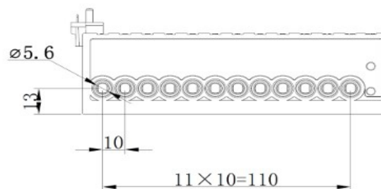
Měřič CT nebo CTPT (jednotka: mm)
