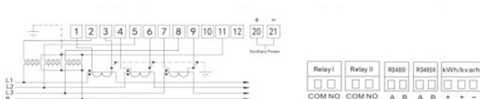
Třífázové, čtyřvodičové, připojené přes transformátory napětí a proudu
